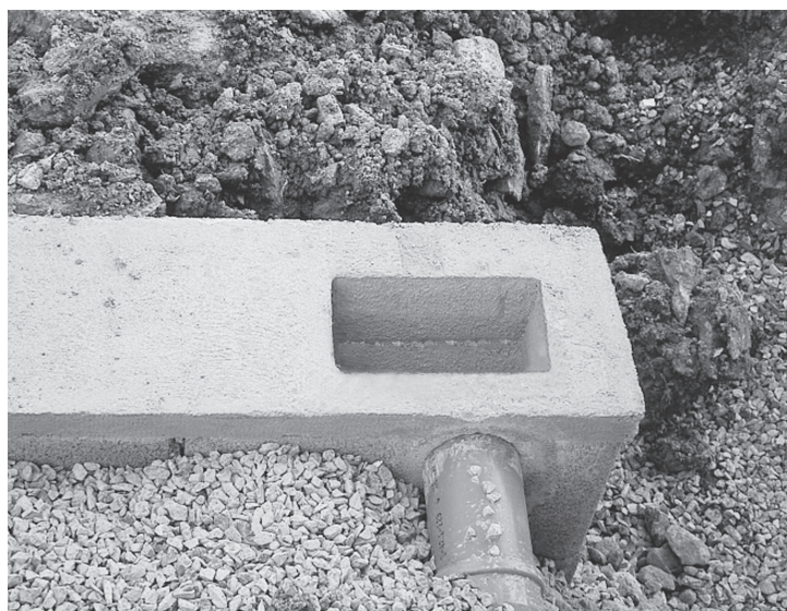
Illustr. à droite: Fondation sous la paroi arrière du garage avec ouverture et tuyau d'écoulement (ici, guidé vers l'avant)
